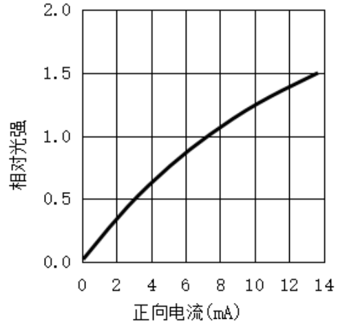
正向电流与相对光强特性曲线
